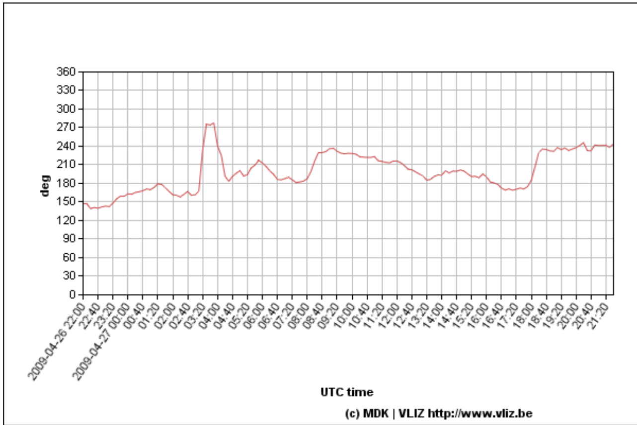
significante golfhoogte gemeten ter hoogte van de Westhinder om de 30 minuten
